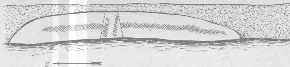
Рис. 1. Джиалский грот (разрез)
