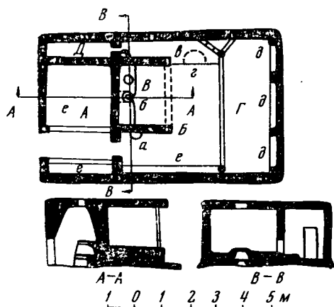
Рис. 4. План и разрезы восточного варианта позднего традиционного жилища. Дом Рахматулаева Х., к. Маргиб (Фан); А — веранда — айвон, Б — прихожая — кучаги; В — очажное отделение — мур; Г — чистое отделение — пасти боло; Д — кладовая — қазнок; а — яма-зернохранилище — чагора; б — очаг; в — возвышение для стряпни — ошхона; г — ниша для дров в толще возвышения ошхоны; д — стенные ниши — ток; е — глинобитное возвышение — суфа
