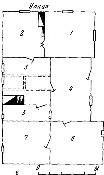
Рис. 5. Дом рабочего совхоза Я. Шнайдера в селе Октябрьское Карасукского района, построенный в 1954 г. а — внешний вид; б — план; 1 — жилая комната, 2 — кухня, 3 — кухня-столовая, 4 — сени, 5 — кладовая, 6 — коровник, 7 — сеник (дровяник)
