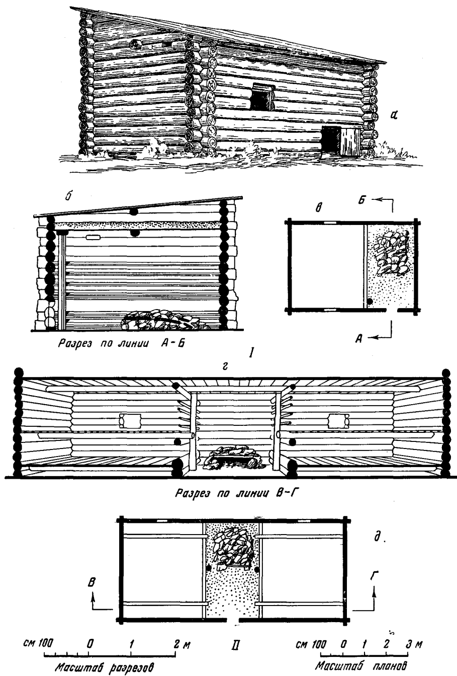
Рис. 9. Риги Братского района: I — односадная рига, д. Наратаи: а — общий вид, б — разрез, в — план; II — двухсадная рига, д. Романово: з — разрез, д — план
