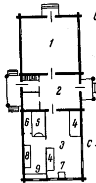
Рис 5. Старинный дом «связью», д. Громы Братского района: а — внешний вид; б — наличники окна задней избы; в — план: 1 — передняя изба (ныне занята под магазин), 2 — сени, 3 — задняя изба, 4 — кровать, 5 — печь, 6 — голбец, 7 — стол, 8 — курятник, 9 — лавка; г — повал
