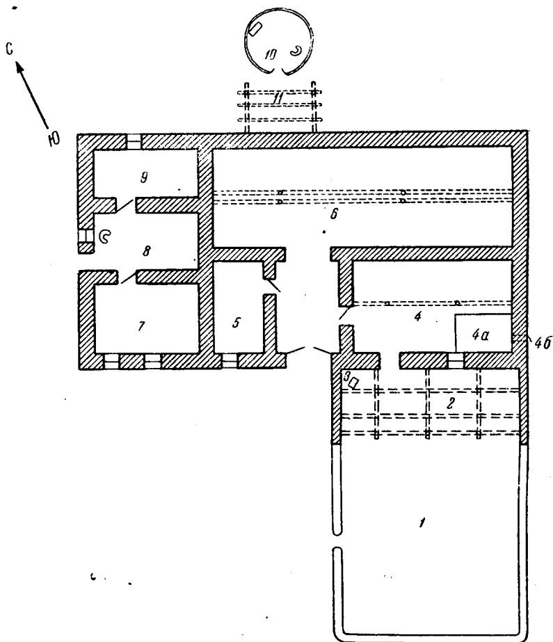
Рис. 5. План хозяйственных построек 11-й бригады колхоза им. Ахунбаева: 1 — открытая площадка для просушки хлопка, собранного на полях бригады; 2 — навес (шертек); 3 — десятичные весы; 4 — хлопковый склад с обогреваемой снизу суфой (4а) для просушки хлопка в плохую погоду; 4б — топка для нагрева суфы; 5 — второе помещение хлопкового склада; 6 — хлев (сеисхона) для рабочего скота бригады; 7 — кладовая для сельскохозяйственного инвентаря и другого имущества бригады; 8 — хозяйственное помещение с очагом; 9 — комната сторожа; 10 — юрта сторожа; 11 — навес (шертек)
